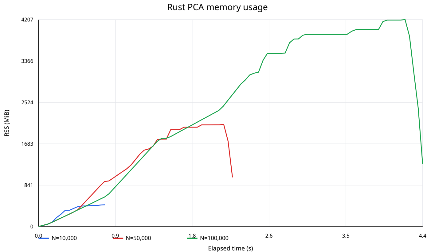
Figure 2: PCA-only RSS
