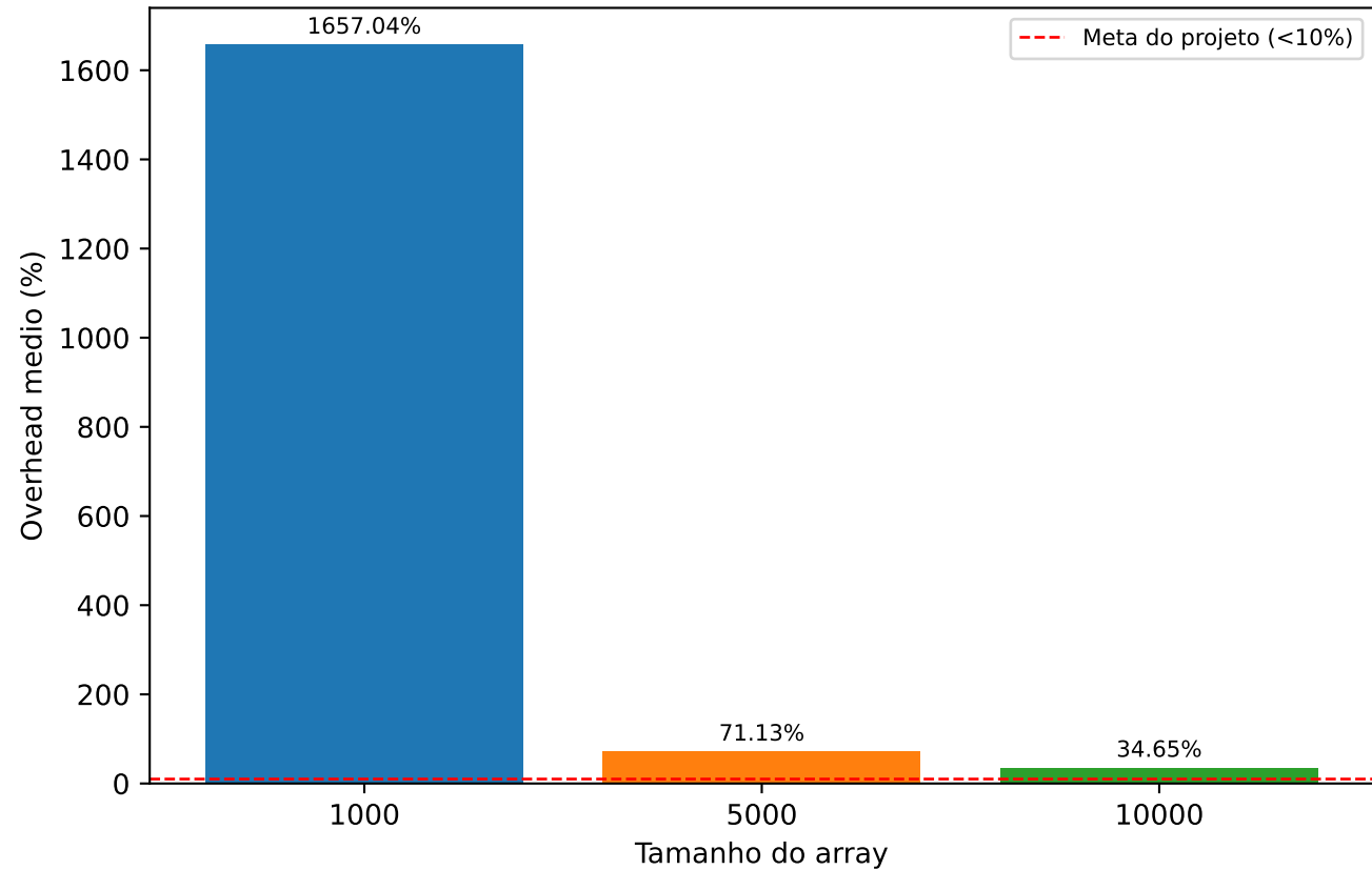
Overhead medio do seletor por tamanho de array (media geral: 587.61%)
