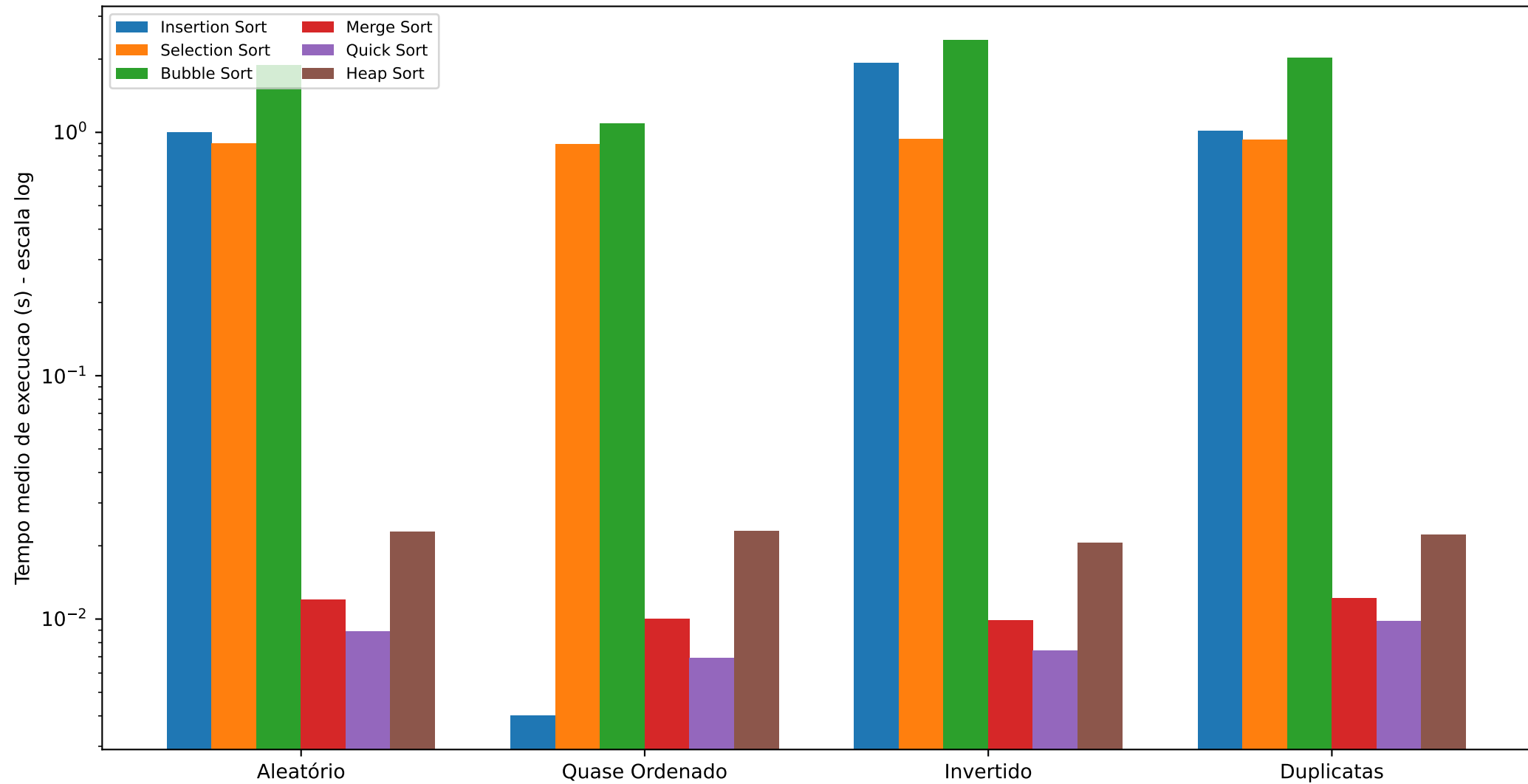
Comportamento dos algoritmos por tipo de conjunto de dados
