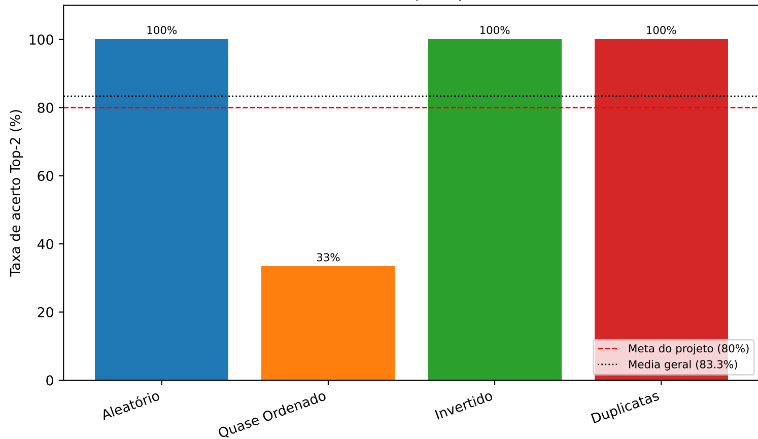
Acuracia do seletor por tipo de dataset
