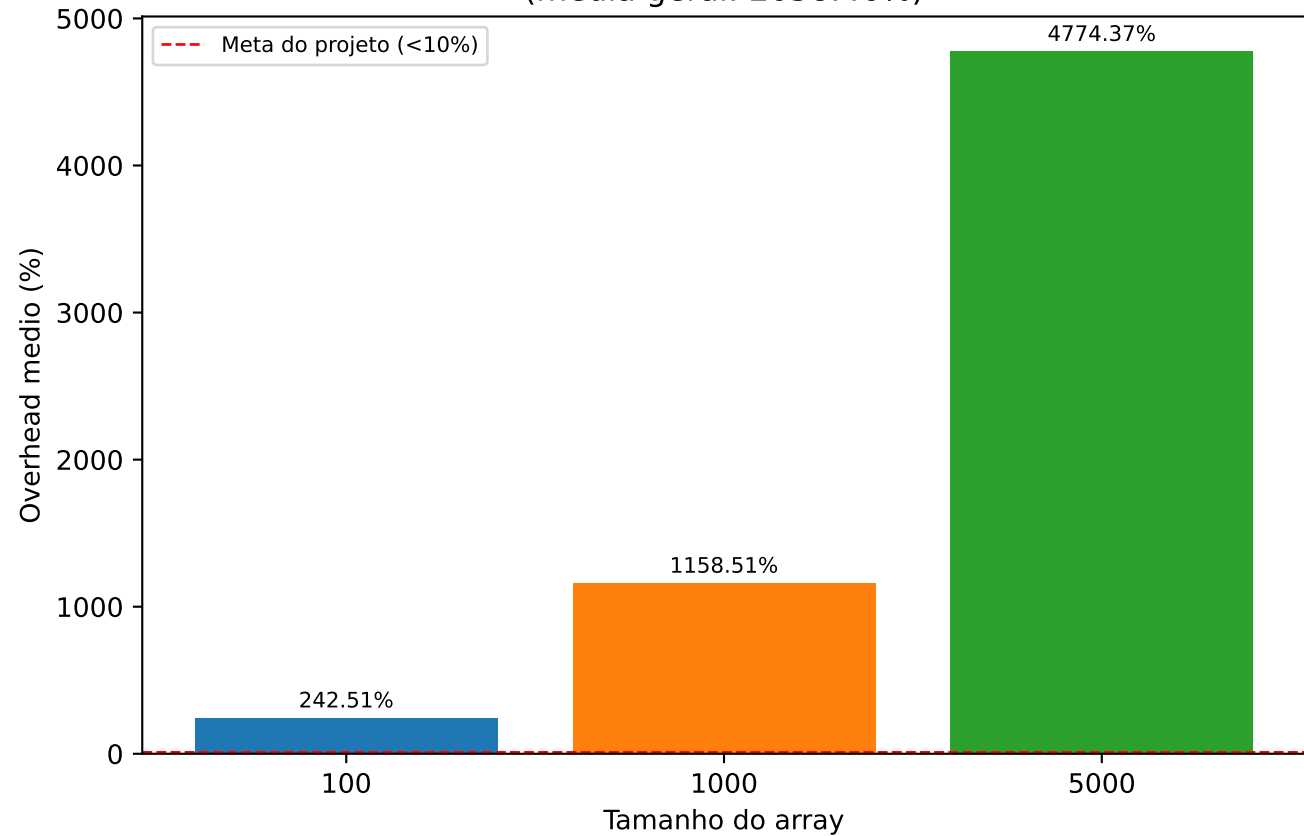
Overhead medio do seletor por tamanho de array (media geral: 2058.46%)
