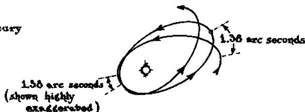
MERCURY'S ACTUAL ORBIT
