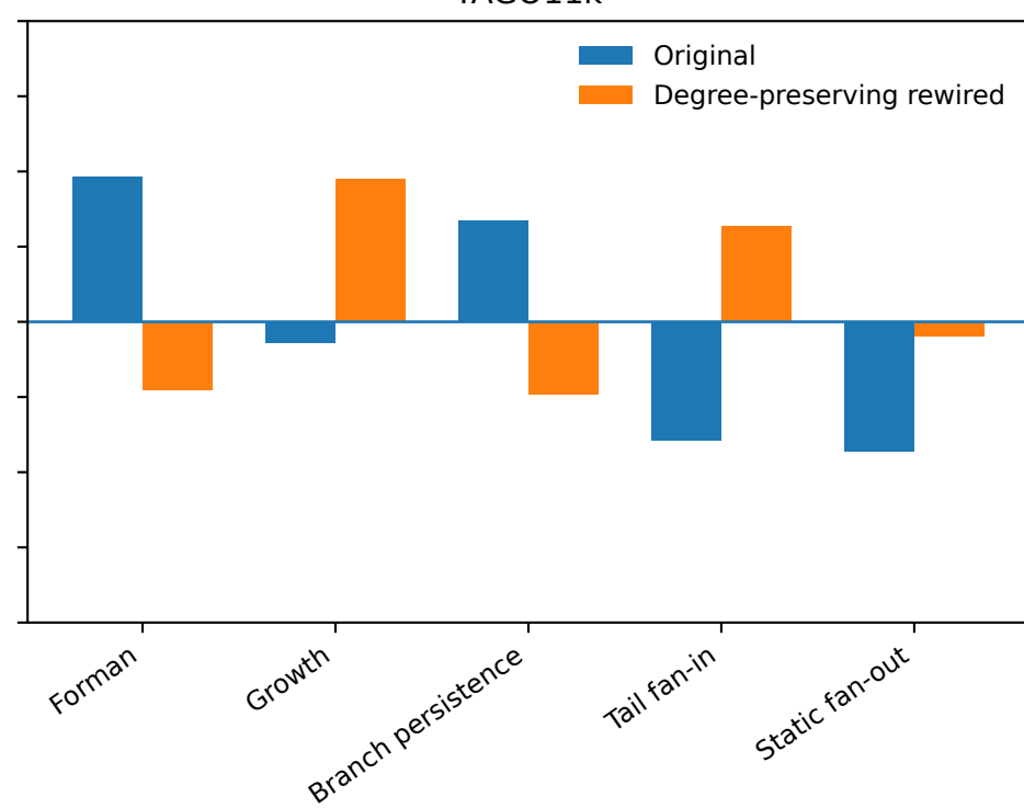
YAGO11k
