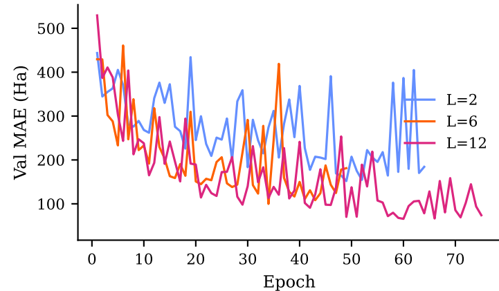
GCN
