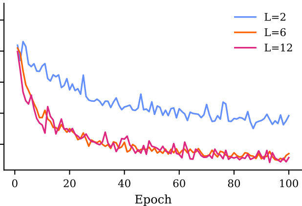
GATv2
