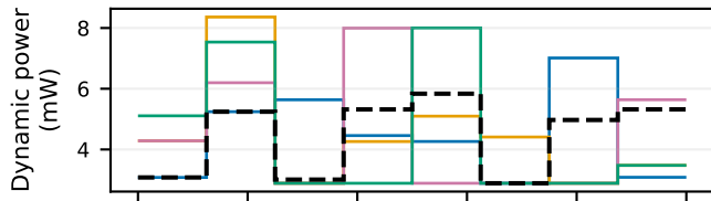
DMA / random_300
