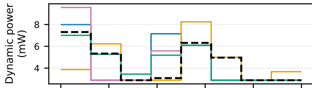
DMA / random_301
