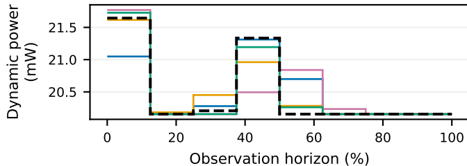
DMA / random_301
