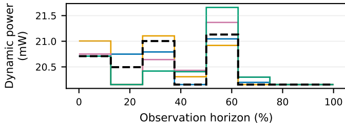
DMA / random_300
