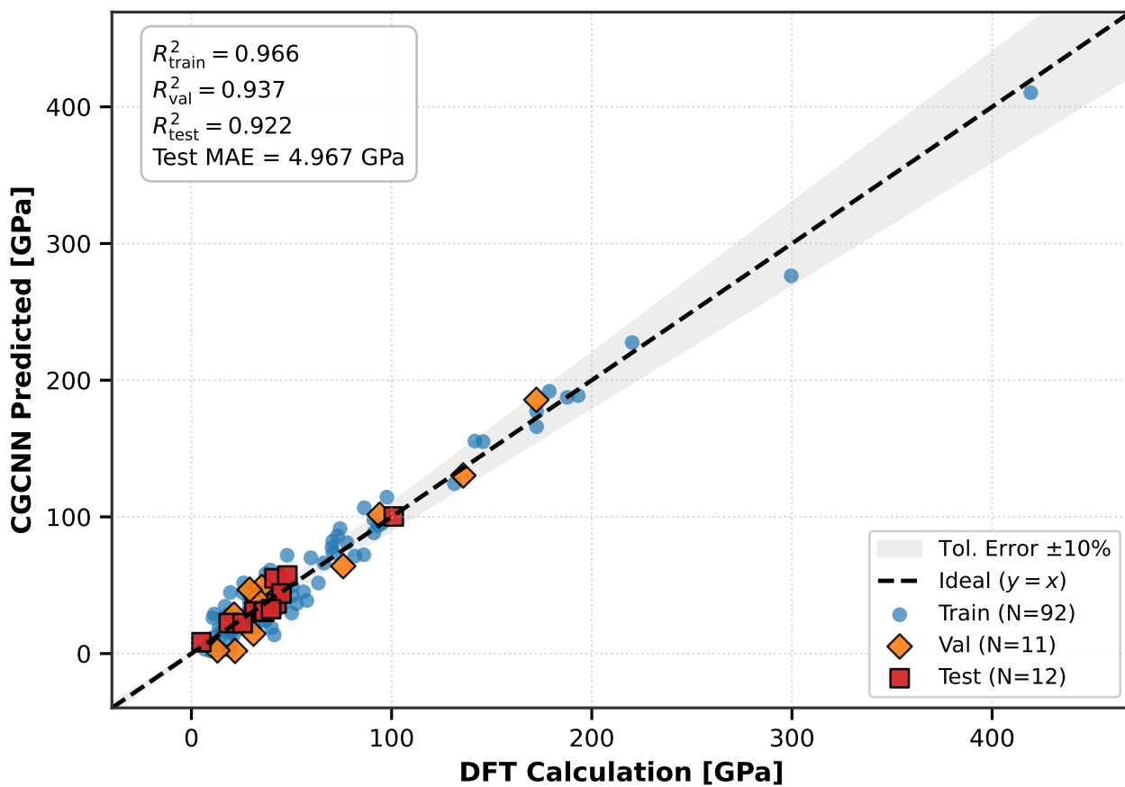
(d) Bulk Modulus ( K )
