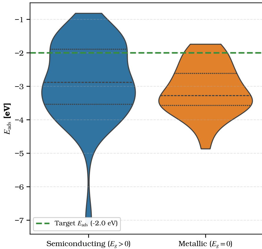
(d) Li Adsorption Energy Distribution
