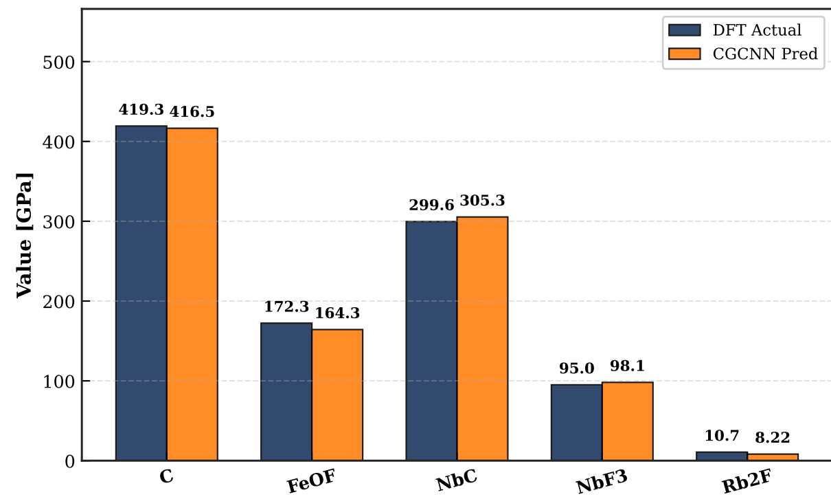
(d) Bulk Modulus ( K )
