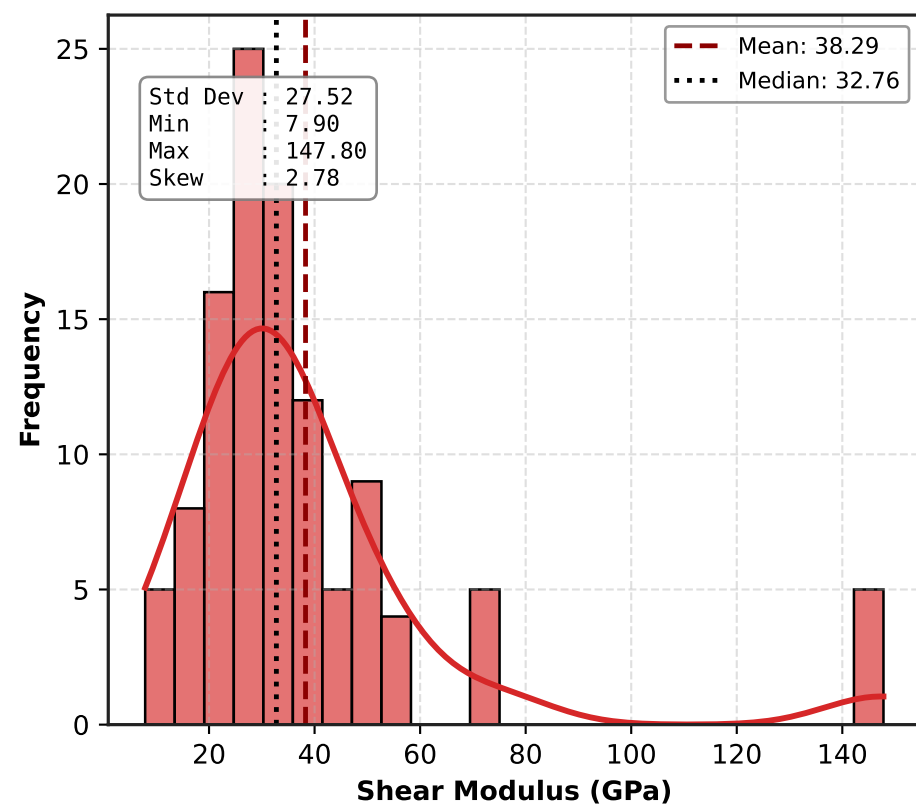
(d) Distribution of Shear Modulus (GPa)
