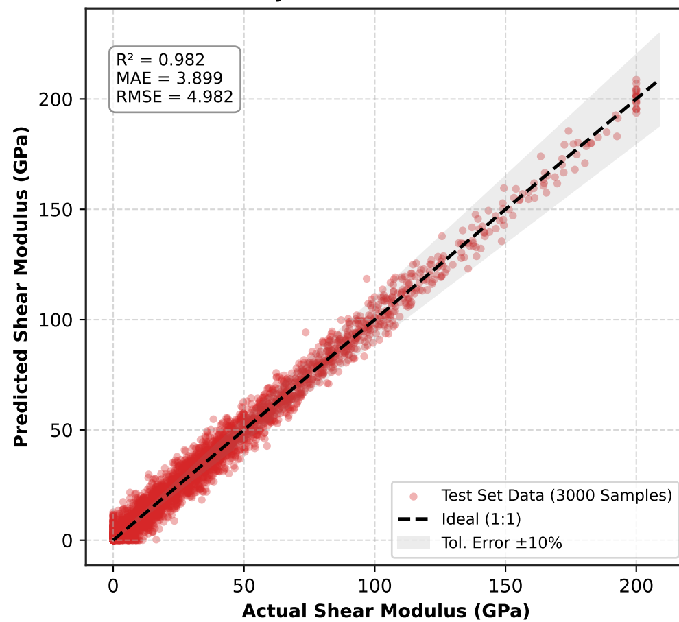
(d) Parity Plot: Shear Modulus (GPa)
