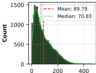
(d) Bulk Modulus (GPa)
