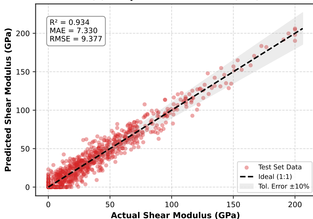
(d) Parity Plot: Shear Modulus (GPa)
