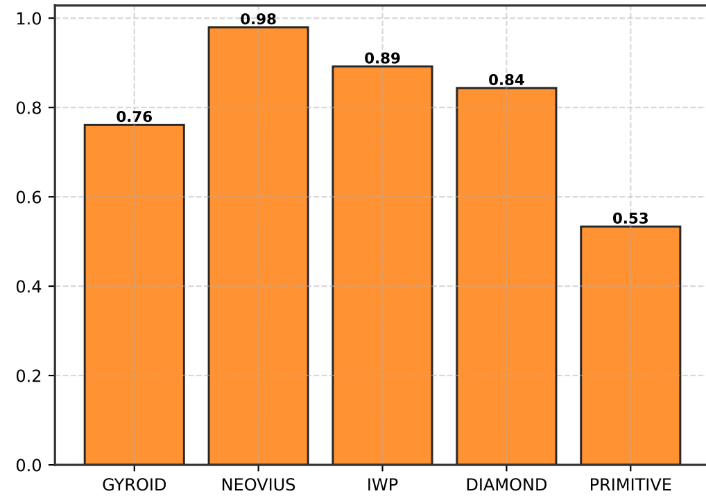
(d) Shear Modulus (GPa) [Shear Strength]
