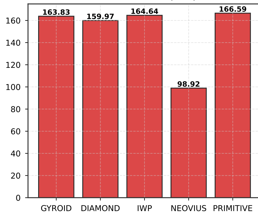
Shear Modulus (GPa)
