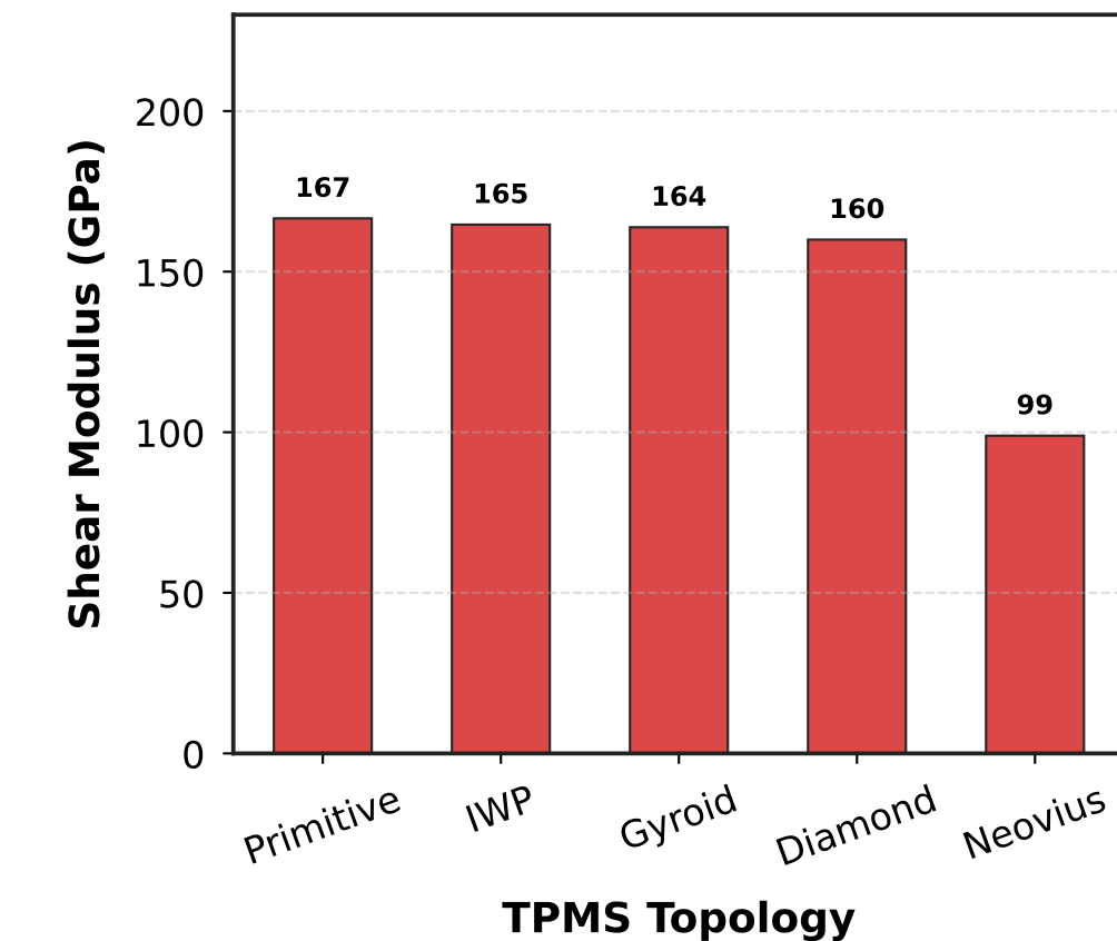
TPMS Topology (d) Shear Modulus (GPa)
