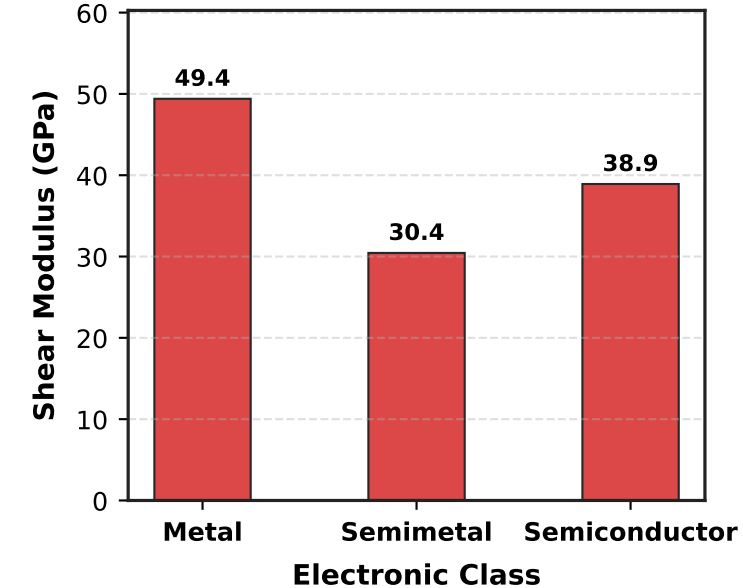
(d) Mean Shear Modulus (GPa)
