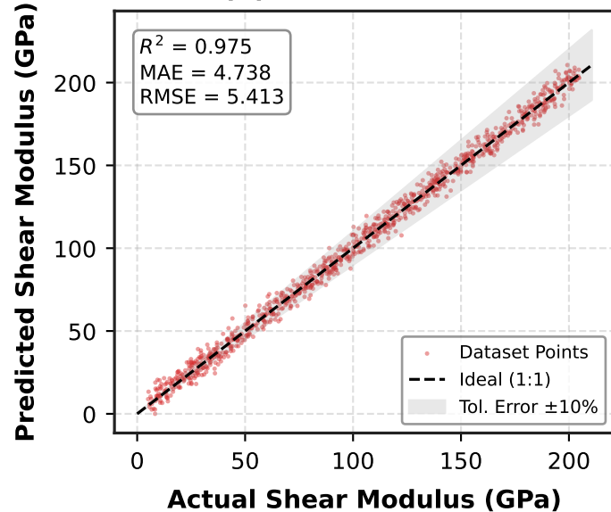
(d) Shear Modulus
