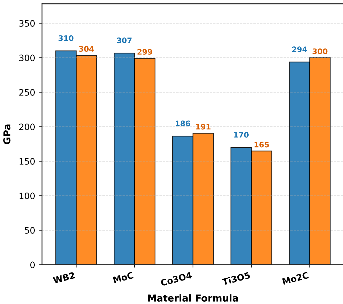
(c) Bulk Modulus (GPa)
