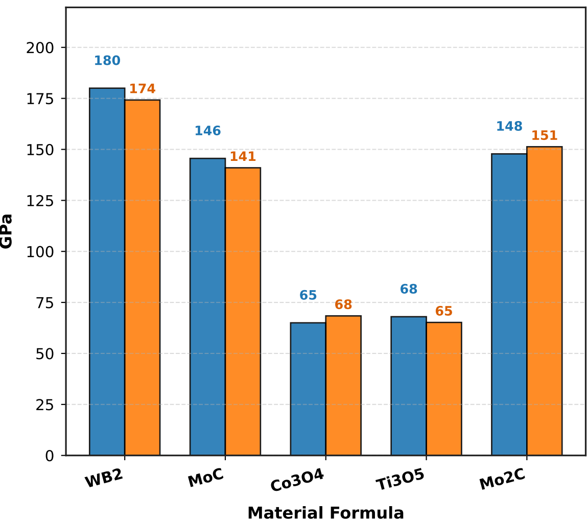
(d) Shear Modulus (GPa)
