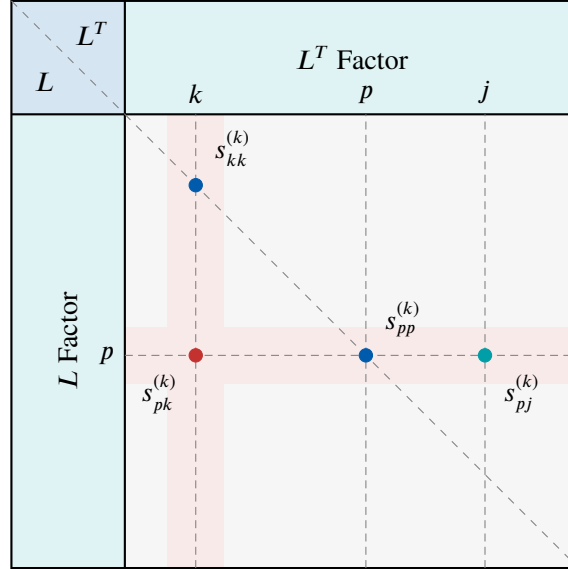
图 3.5 Bunch–Kaufman 选主元
