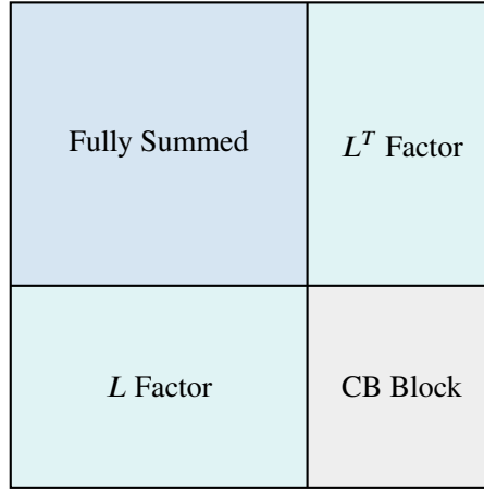
图 3.4 对称超节点对应的波前矩阵。
