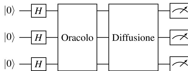
Figura 4.1: Schema dell'algoritmo di Grover su tre qubit. Il blocco oracolo + diffusione viene ripetuto circa \frac{\pi}{4}\sqrt{N} volte prima della misura.
