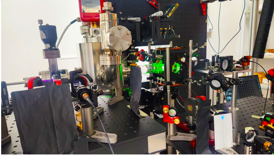
Figura 3.3: Il banco ottico della piattaforma ad atomi neutri del CNR a Sesto Fiorentino, con la camera a vuoto, le ottiche e i fasci laser. Fonte: ICSC / CNR.
