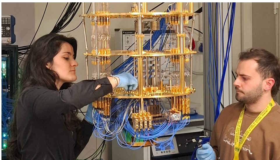
Figura 3.1: Ricercatori del Dipartimento di Fisica Ettore Pancini al lavoro sul criostato di Partenope durante l'installazione del nuovo processore a 64 qubit (2026). Fonte: ICSC.
