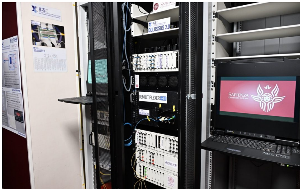
Figura 3.2: I rack di Qolossus 2.0 alla Sapienza, con i moduli fotonici etichettati Qolossus 2.0 , CNR-IFN e Demultiplexer . Fonte: Sapienza Università di Roma / ICSC.
