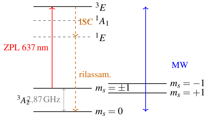
Figura 2.2: Struttura dei livelli energetici del centro \text{NV}^- . La transizione ottica a 637 nm (ZPL, zero-phonon line ) eccita il tripletto; il inter-system crossing (ISC) verso il singoletto ^1A_1 pompa preferenzialmente la popolazione in m_s = 0 , abilitando l'inizializzazione ottica del qubit.
