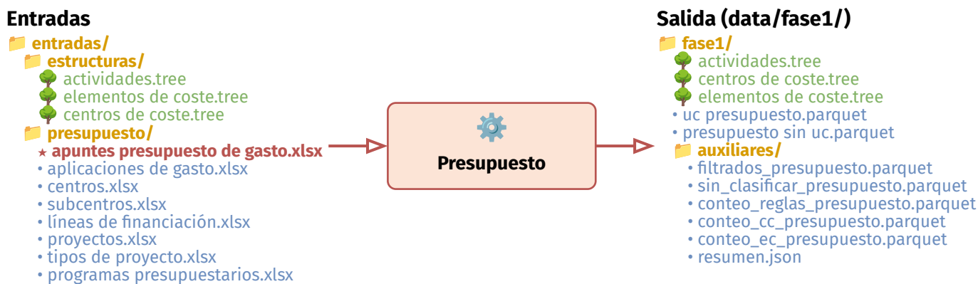
Figura 2: Etapa de presupuesto: ficheros de entrada y salidas que produce.
