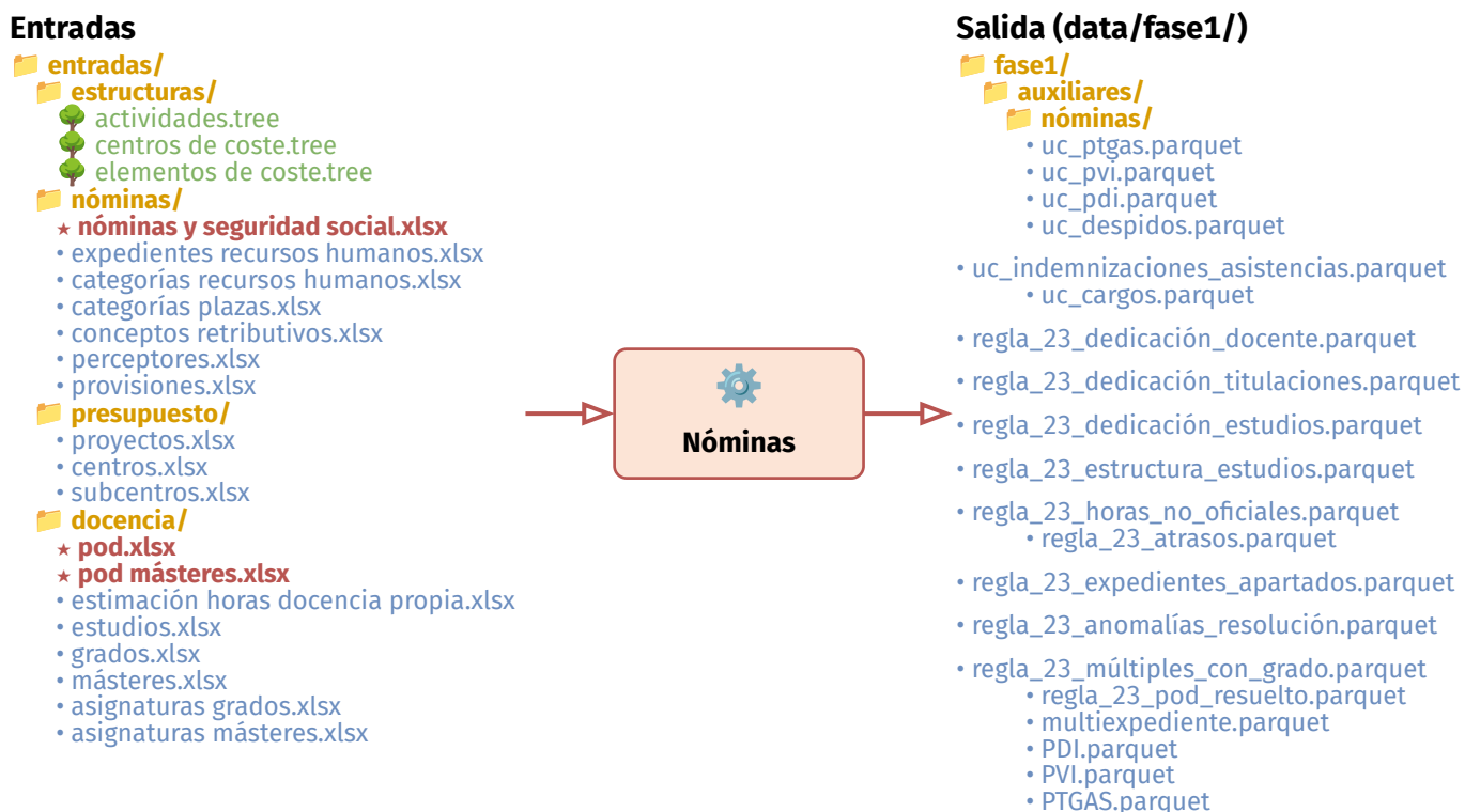
Figura 6: Etapa de nóminas: ficheros de entrada y salidas que produce.
