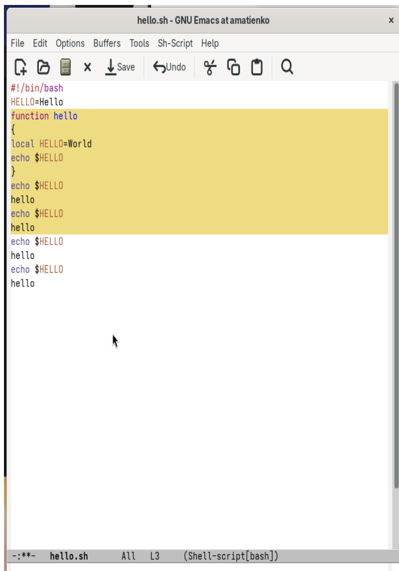
Рисунок 2.4: Выделение блока
