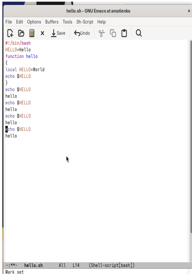
Рисунок 2.3: Операция вставка
