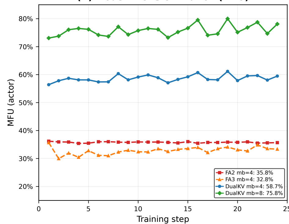
(D) Model FLOPs Utilization (MFU)
