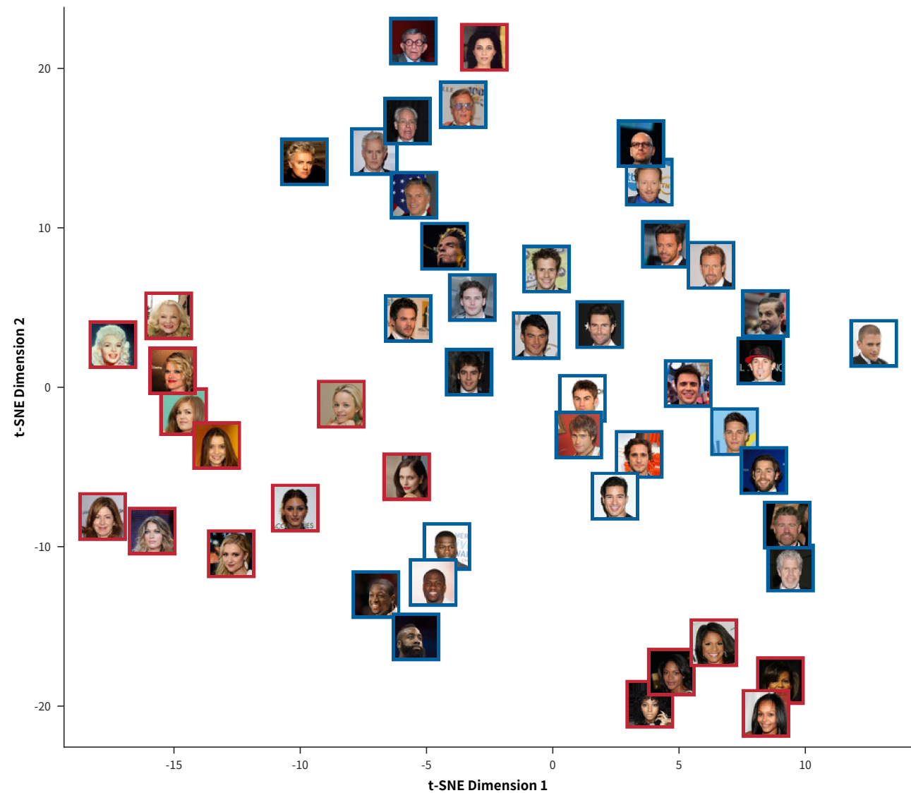
US Visual Embedding t-SNE
