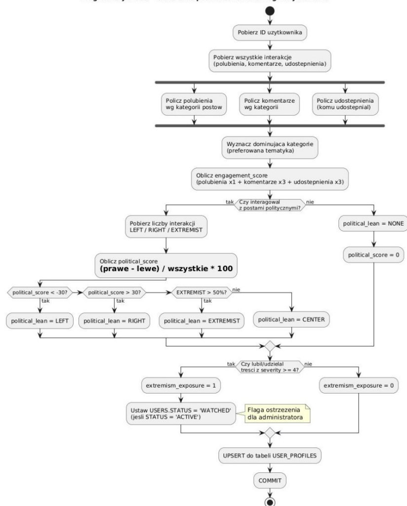
Diagram czynności - Obliczanie profilu behawioralnego użytkownika
