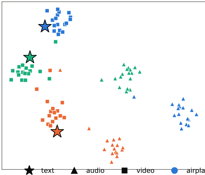
SCA (ours)
