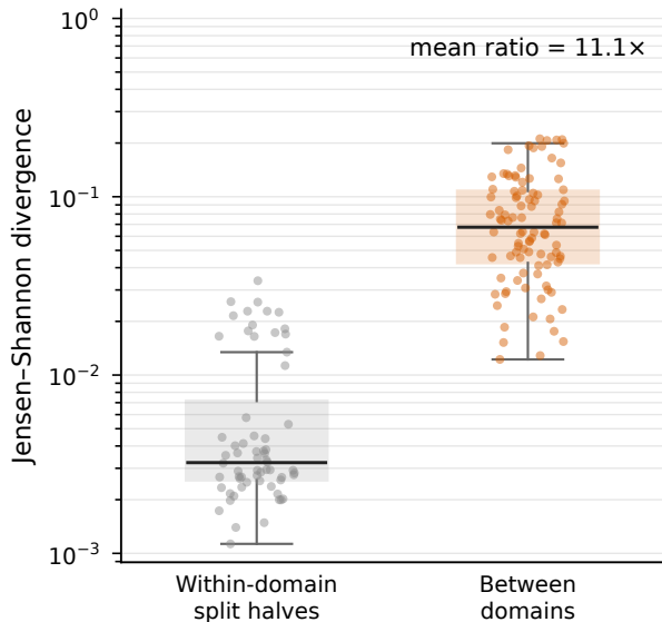
(a) Prefill
