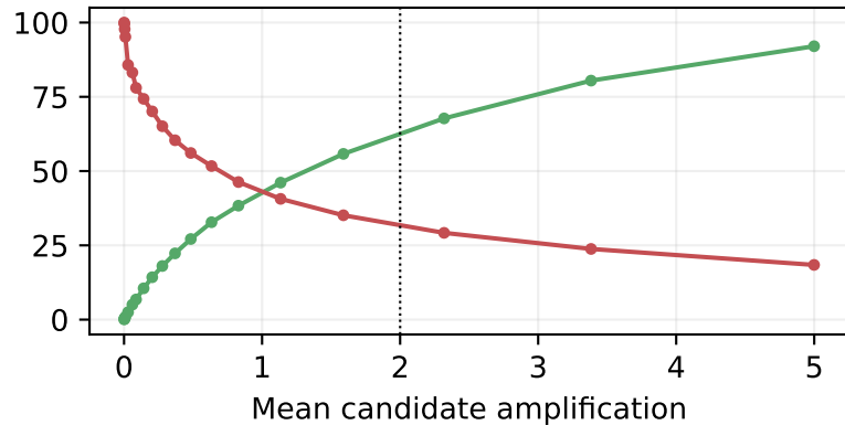
Decode \Delta=1
