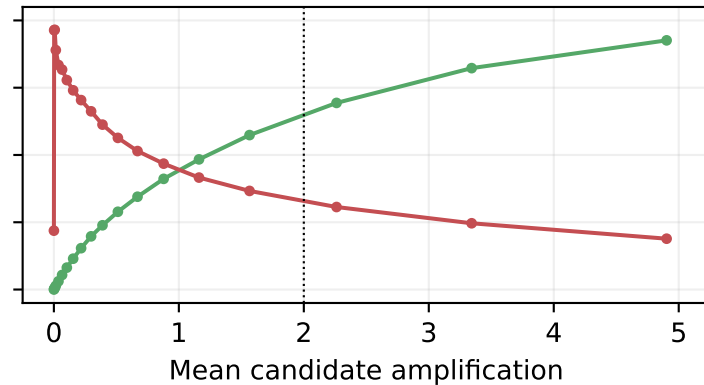
Decode \Delta=3
