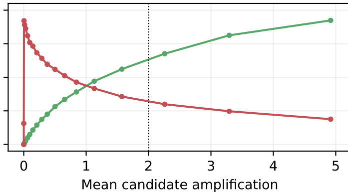
Decode \Delta=2
