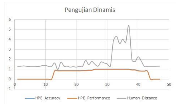
Gambar 17. Hasil grafik pengujian dinamis
