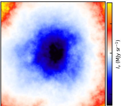
070 \mu\text{m} , 8.4 arcsec
