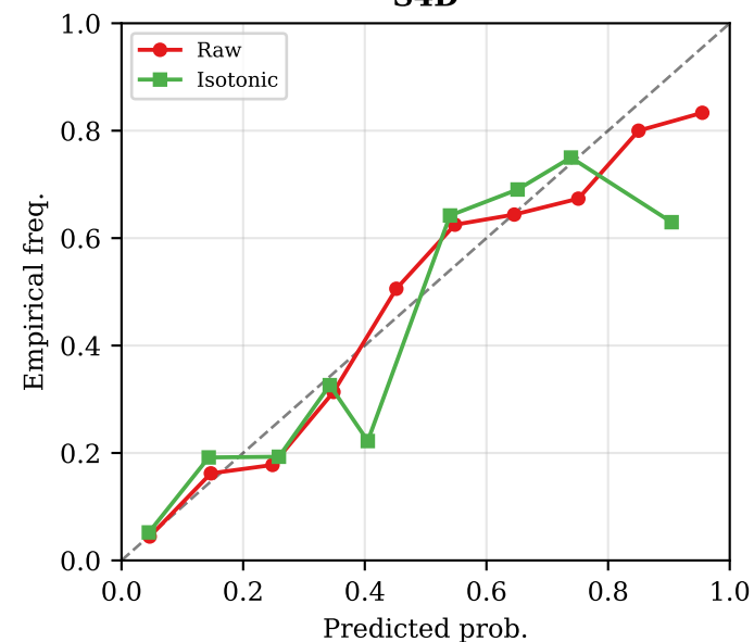
S4D
