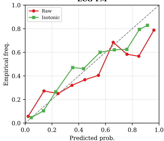
ECG-FM
