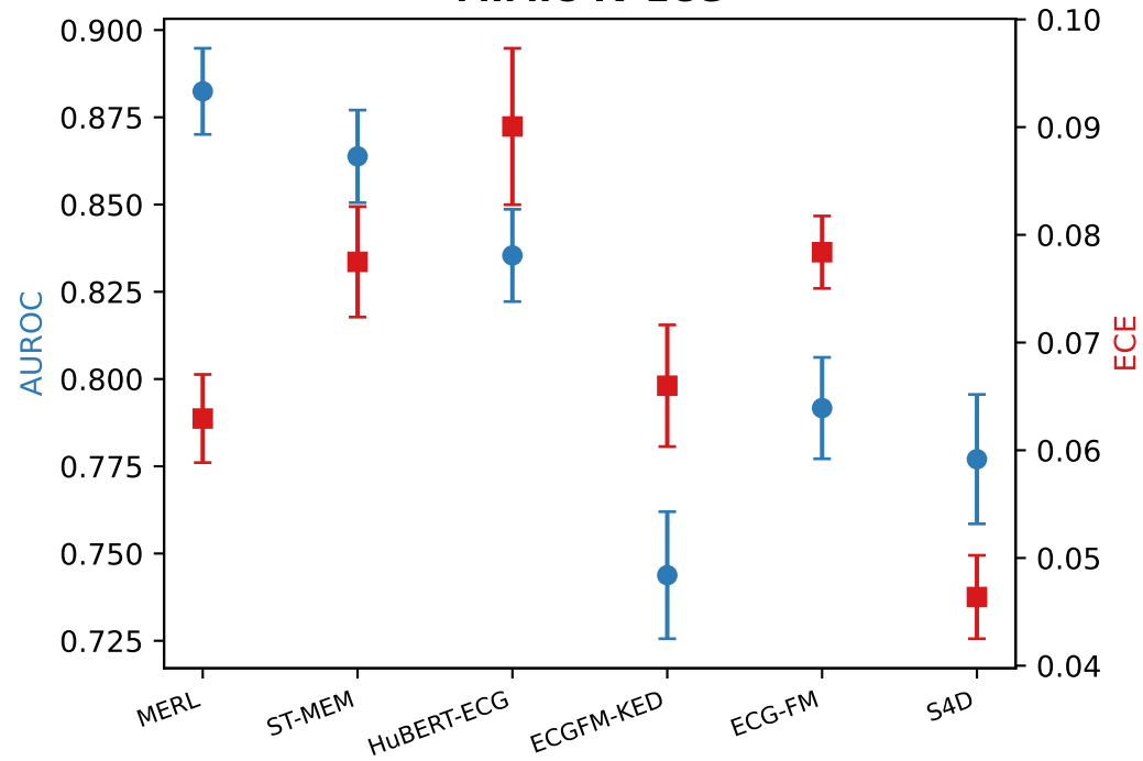
MIMIC-IV-ECG
