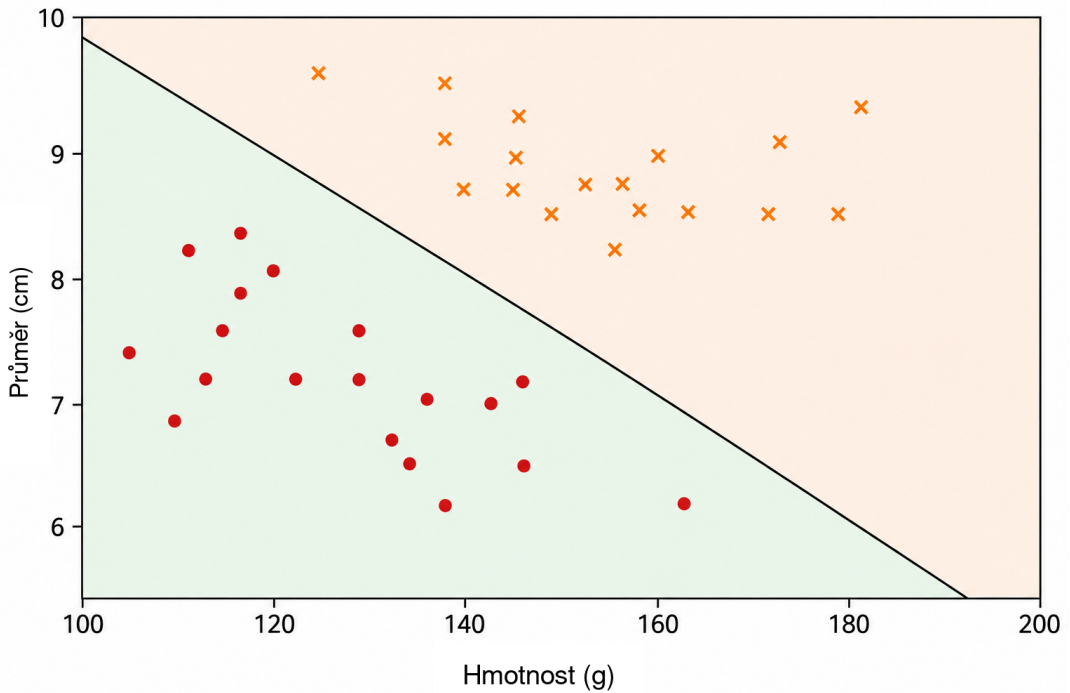
Obrázek 2: Příklad lineárního klasifikátoru v rovině hmotnost–průměr. Přímka slouží jako rozhodovací hranice: body v jedné polorovině dostanou jednu třídu a body v opačné polorovině druhou. Rozhodnutí tedy závisí pouze na tom, na které straně přímky bod leží.
