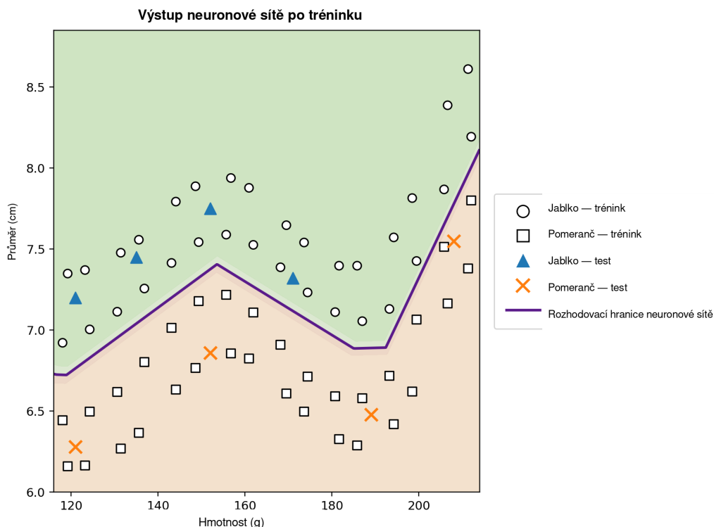
Obrázek 7: Výsledek programu v Pythonu po tréninku neuronové sítě. Syntetický datový soubor obsahuje 64 trénovacích příkladů rozmístěných v široké oblasti roviny hmotnost–průměr a osm dalších příkladů určených k ilustračnímu testu. Zvýrazněná křivka je vrstevnice \hat{y} = 0.5 a představuje naučenou rozhodovací hranici; stínované oblasti ukazují třídy predikované sítí. Kružnice označují trénovací jablka, čtverce trénovací pomeranče, trojúhelníky testovací jablka a křížky testovací pomeranče.
