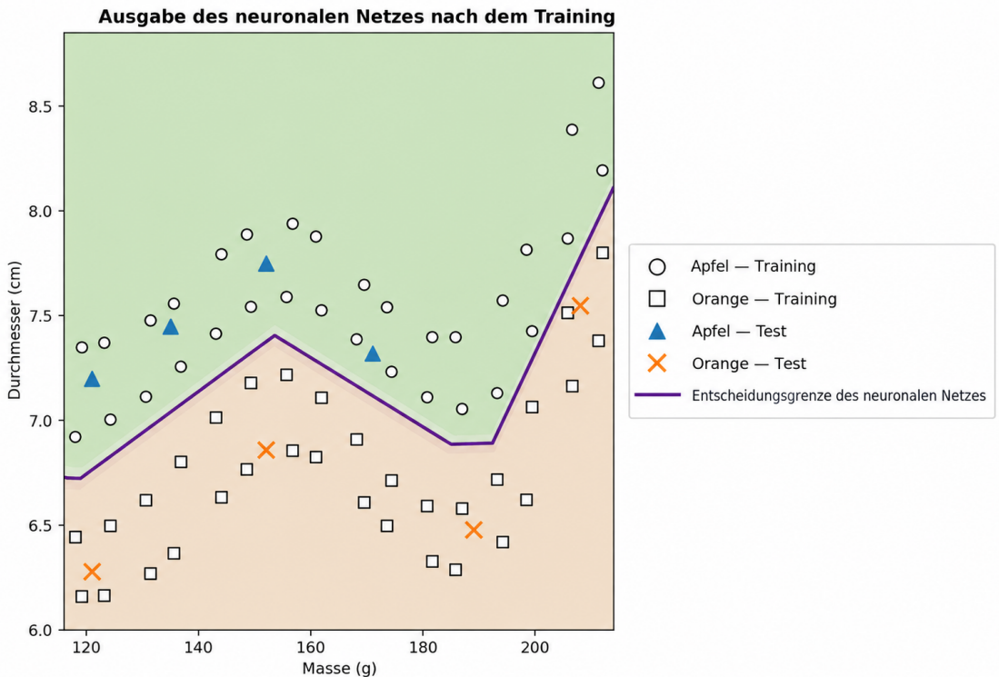
Abbildung 7: Python-Ausgabe nach dem Training des neuronalen Netzes. Der synthetische Datensatz enthält 64 Trainingsbeispiele, die über einen großen Bereich der Masse–Durchmesser-Ebene verteilt sind, sowie acht zusätzliche Beispiele für einen illustrativen Test. Die hervorgehobene Kurve ist das Niveau \hat{y} = 0.5 und stellt die gelernte Entscheidungsgrenze dar; die schattierten Bereiche zeigen die vom Netz vorhergesagten Klassen. Kreise repräsentieren Trainingsäpfel, Quadrate Trainingsorangen, Dreiecke Testäpfel und Kreuze Testorangen.
