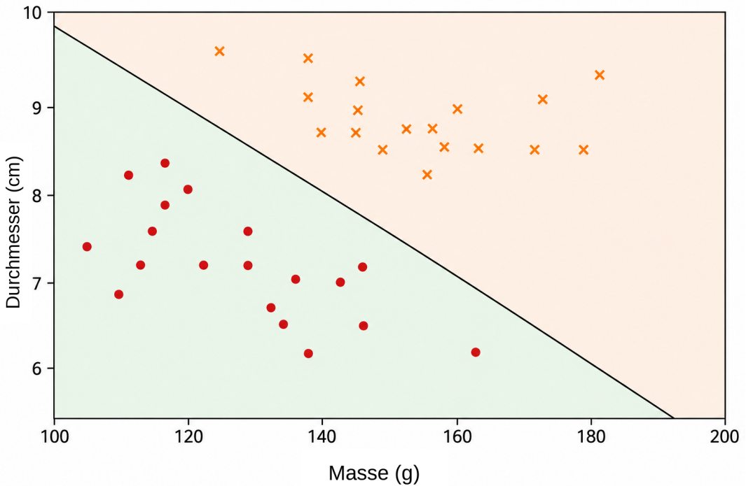
Abbildung 2: Beispiel eines linearen Klassifikators in der Masse–Durchmesser-Ebene. Die Gerade dient als Entscheidungsgrenze: Punkte in einer Halbebene erhalten die eine Klasse, Punkte in der gegenüberliegenden Halbebene die andere. Die Entscheidung hängt somit ausschließlich davon ab, auf welcher Seite der Geraden sich der Punkt befindet.
