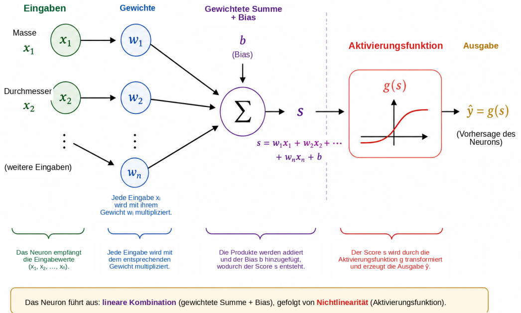
Abbildung 3: Schematische Funktionsweise eines künstlichen Neurons. Jede Eingabe x_i wird mit einem Gewicht w_i multipliziert; die Produkte werden zum Bias b addiert und ergeben den Score s . Die Aktivierungsfunktion g transformiert diesen Score anschließend in die Ausgabe \hat{y} = g(s) , die als Zwischengröße oder als endgültige Vorhersage verwendet werden kann.
