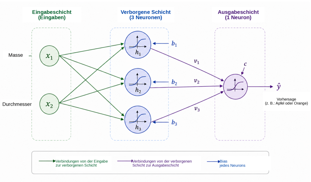
Abbildung 5: Didaktische 2–3–1-Architektur zur Einführung in die Berechnungen neuronaler Netze. Die beiden Eingaben — Masse und Durchmesser — speisen drei Neuronen in der verborgenen Schicht. Deren Aktivierungen h_1, h_2, h_3 werden anschließend vom Ausgabeneuron kombiniert, um die Vorhersage \hat{y} zu erzeugen. Jede Verbindung besitzt ein anpassbares Gewicht, und jedes Neuron besitzt einen Bias.
