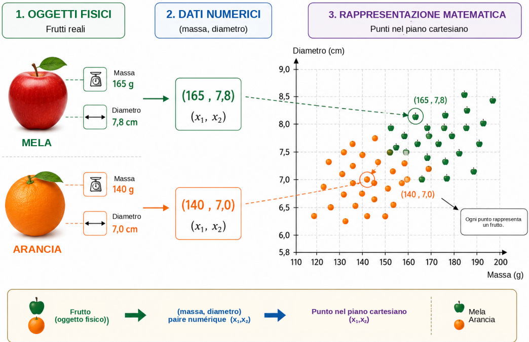
Figura 1: Dall'osservazione fisica alla modellizzazione matematica. Ogni frutto viene prima descritto mediante due grandezze misurabili — massa e diametro — e quindi rappresentato dalla coppia ordinata (x_1, x_2) . Nel piano massa–diametro, ogni osservazione diventa un punto, così che distinguere le mele dalle arance può essere reinterpretato come un problema geometrico di separazione di due classi.
