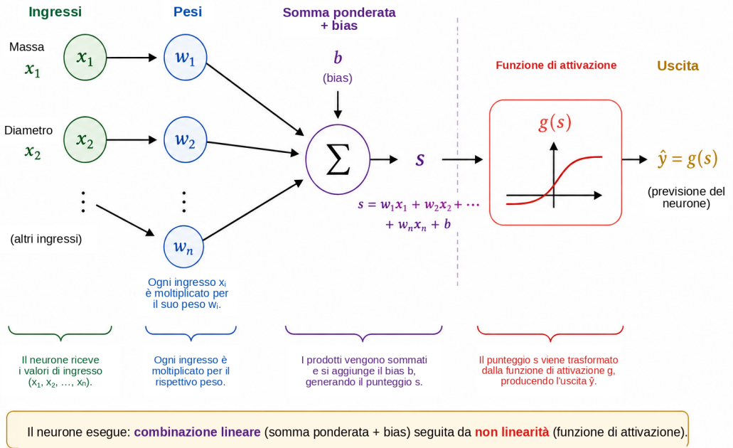
Figura 3: Funzionamento schematico di un neurone artificiale. Ogni ingresso x_i viene moltiplicato per un peso w_i ; i prodotti vengono sommati al bias b per produrre il punteggio s . La funzione di attivazione g trasforma quindi questo punteggio nell'uscita \hat{y} = g(s) , che può essere utilizzata come quantità intermedia o come previsione finale.
