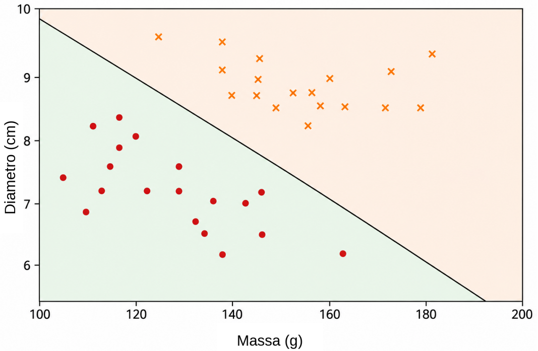
Figura 2: Esempio di classificatore lineare nel piano massa–diametro. La retta svolge il ruolo di frontiera di decisione: i punti di un semipiano ricevono una classe, mentre quelli del semipiano opposto ricevono l'altra. La decisione dipende quindi unicamente dal lato della retta in cui si trova il punto.
