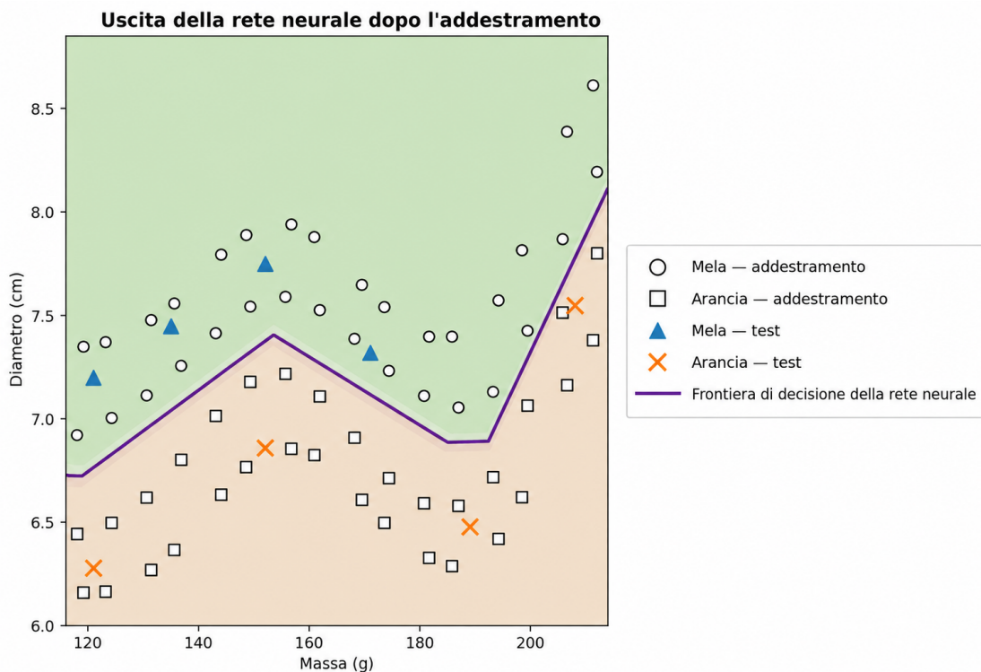
Figura 7: Uscita di Python dopo l'addestramento della rete neurale. L'insieme di dati sintetico contiene 64 esempi di addestramento distribuiti su un'ampia regione del piano massa–diametro e otto esempi aggiuntivi riservati a un test illustrativo. La curva evidenziata corrisponde al livello \hat{y} = 0.5 e rappresenta la frontiera di decisione appresa; le regioni ombreggiate indicano le classi previste dalla rete. I cerchi rappresentano le mele di addestramento, i quadrati le arance di addestramento, i triangoli le mele di test e le croci le arance di test.
