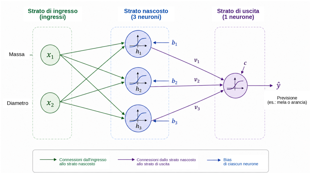
Figura 5: Architettura didattica 2–3–1 utilizzata per introdurre il calcolo in una rete neurale. I due ingressi — massa e diametro — alimentano tre neuroni dello strato nascosto. Le loro attivazioni h_1, h_2, h_3 vengono poi combinate dal neurone di uscita per produrre la previsione \hat{y} . Ogni connessione possiede un peso regolabile e ogni neurone ha un bias.
