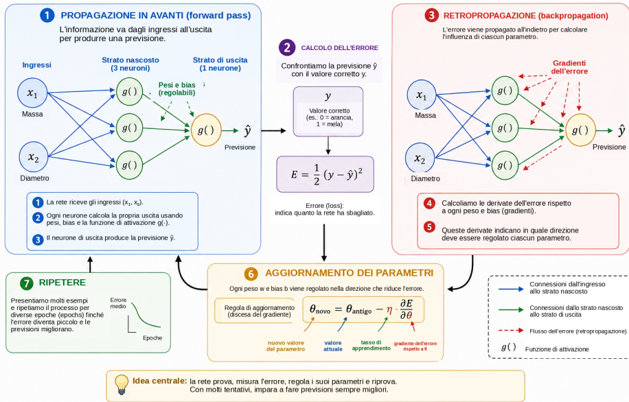
Figura 6: Ciclo fondamentale di addestramento di una rete neurale. Il passaggio in avanti trasforma gli ingressi in una previsione; la funzione di perdita misura la discrepanza tra la previsione e l'obiettivo; la retropropagazione calcola i gradienti mediante la regola della catena; e la discesa del gradiente utilizza tali gradienti per aggiornare pesi e bias. Ripetere questo ciclo per molte epoche è ciò che chiamiamo apprendimento.
