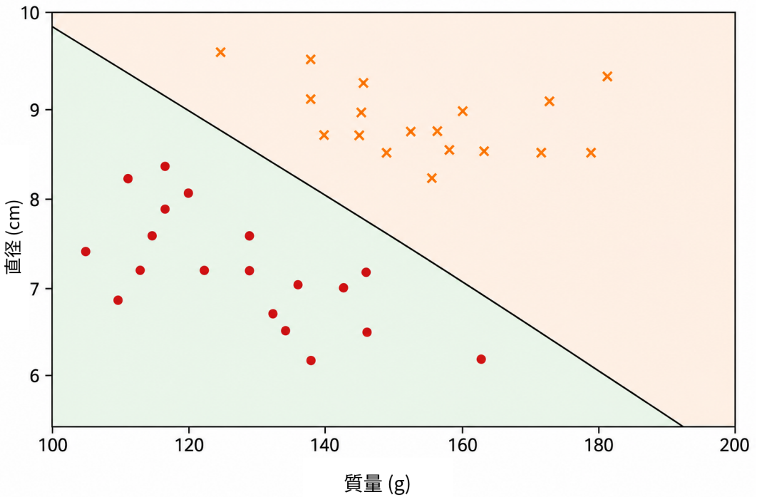
図 2: 質量-直径平面における線形分類器の例。直線は決定境界として働き，一方の半平面にある点には一つのクラスが，他方の半平面にある点には別のクラスが割り当てられる。したがって判断は，点が直線のどちら側にあるかだけで決まる。
