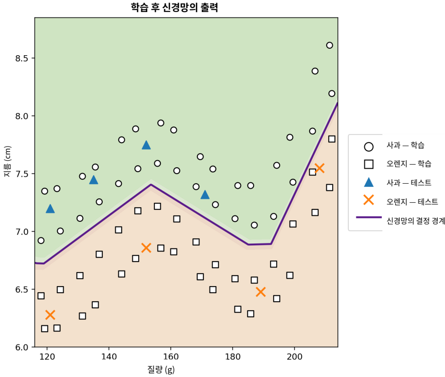
그림 7: 신경망 학습 후 얻은 Python 출력. 합성 데이터 집합에는 질량-지름 평면의 넓은 영역에 분포한 64 개의 학습 예제와 설명용 테스트로 별도 확보한 8 개의 예제가 포함된다. 강조된 곡선은 \hat{y} = 0.5 등고선이며 학습된 결정 경계를 나타낸다. 색 영역은 네트워크가 예측하는 클래스를 보여 준다. 원은 학습용 사과, 사각형은 학습용 오렌지, 삼각형은 테스트용 사과, × 표시는 테스트용 오렌지를 나타낸다.
