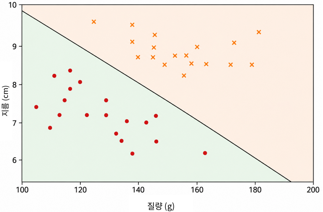
그림 2: 질량-지름 평면에서의 선형 분류기의 예. 직선은 결정 경계로 작용하며, 한 반평면의 점에는 한 클래스가, 다른 반평면의 점에는 다른 클래스가 할당된다. 따라서 판단은 점이 직선의 어느 쪽에 놓이는지만으로 결정된다.
