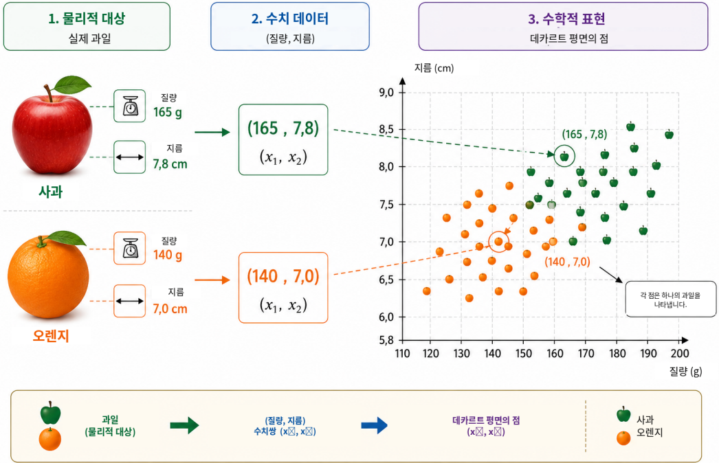
그림 1: 물리적 관찰에서 수학적 모델링으로. 각 과일은 먼저 질량과 지름이라는 두 개의 측정 가능한 양으로 기술되고, 이후 순서쌍 (x_1, x_2) 로 표현된다. 질량-지름 평면에서는 각 관측이 하나의 점이 되므로, 사과와 오렌지를 구별하는 문제를 두 클래스를 분리하는 기하학 문제로 다시 해석할 수 있다.
