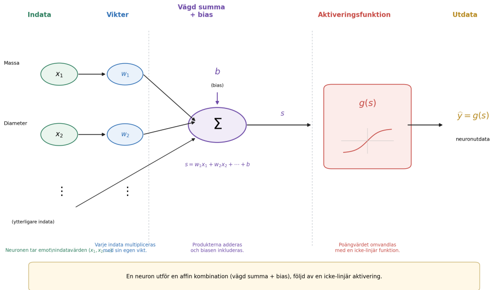
Figur 3: Schematisk funktion hos en artificiell neuron. Varje indata x_i multipliceras med en vikt w_i ; produkterna adderas till biasen b och ger poängvärdet s . Aktiveringsfunktionen g omvandlar därefter detta poängvärde till utdata \hat{y} = g(s) , som kan användas som en mellanliggande storhet eller som den slutliga förutsägelsen.
