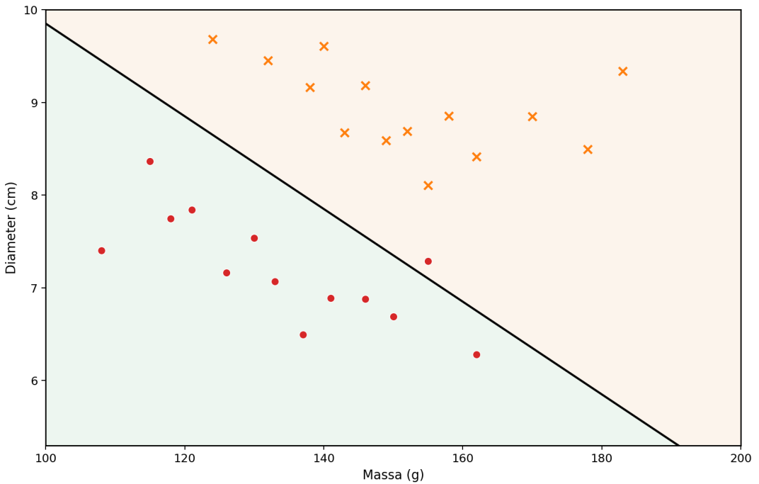
Figur 2: Exempel på en linjär klassificerare i massa–diameter-planet. Den räta linjen fungerar som en beslutsgräns: punkter i det ena halvplanet tilldelas den ena klassen, medan punkter i det motsatta halvplanet tilldelas den andra. Beslutet beror alltså endast på vilken sida av linjen punkten ligger.
