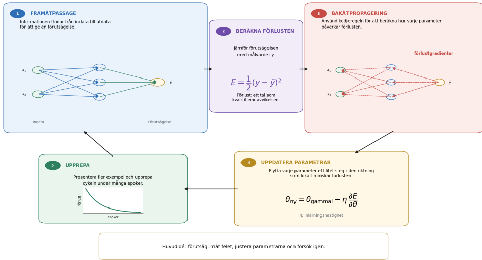
Figur 6: Grundläggande träningscykel för ett neuralt nätverk. Framåtpassagen omvandlar indata till en förutsägelse; förlustfunktionen mäter avvikelser mellan förutsägelse och målvärde; bakåtpropagering beräknar gradienter med kedjeregeln; och gradientnedstigning använder dessa gradienter för att uppdatera vikter och biasparametrar. Att upprepa denna cykel under många epoker är det vi kallar inlärning.
