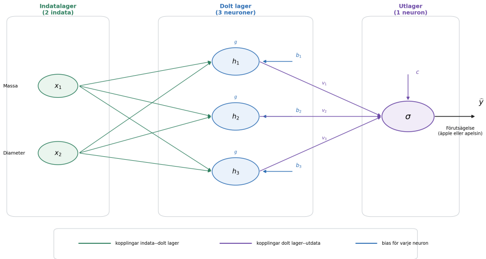
Figur 5: Didaktisk 2–3–1-arkitektur som används för att introducera beräkningar i neurala nätverk. De två indata — massa och diameter — matas till tre neuroner i det dolda lagret. Deras aktiveringar h_1, h_2, h_3 kombineras därefter av utneuronen för att ge förutsägelsen \hat{y} . Varje koppling har en justerbar vikt och varje neuron har en bias.
