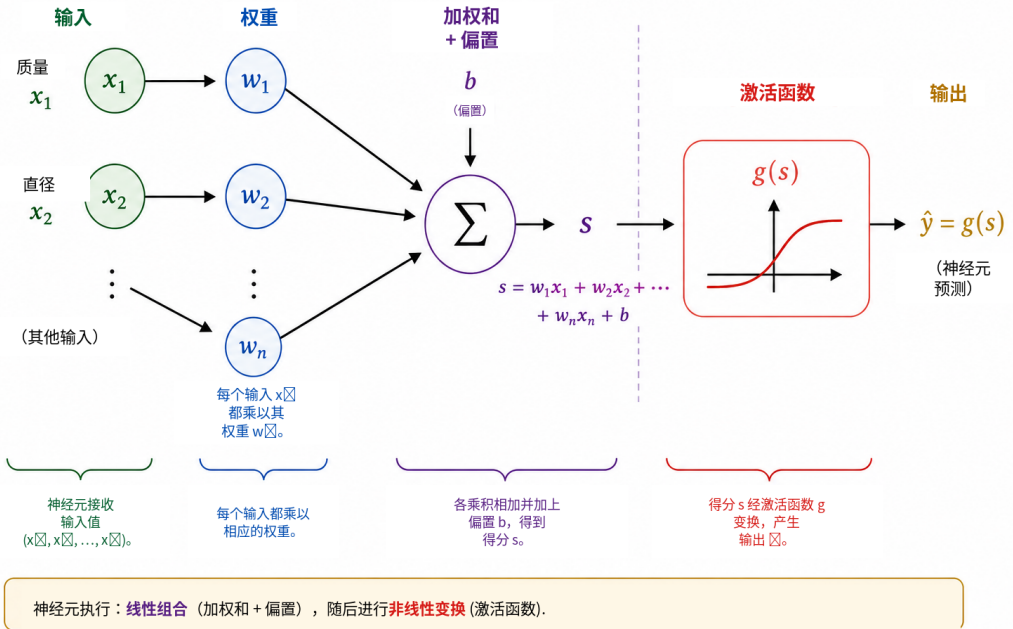
图 3: 人工神经元的示意计算。每个输入 x_i 乘以一个权重 w_i ; 所有乘积与偏置 b 相加, 得到得分 s 。随后激活函数 g 把该得分变换成输出 \hat{y} = g(s) 。这个输出既可以作为网络中的中间量, 也可以作为最终预测。
