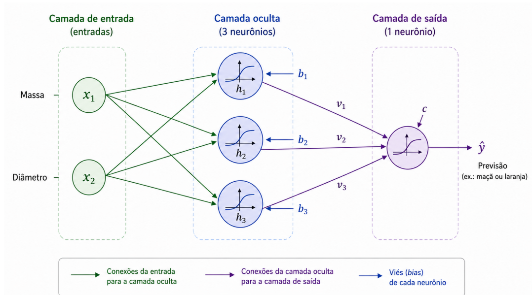
Figura 5: Arquitetura pedagógica 2–3–1 usada para introduzir o funcionamento de uma rede neural. As duas entradas — massa e diâmetro — alimentam três neurônios na camada oculta, cujas ativações h_1 , h_2 , h_3 são combinadas por um neurônio de saída para produzir a previsão \hat{y} . Cada conexão possui um peso ajustável, e cada neurônio possui um viés associado.
