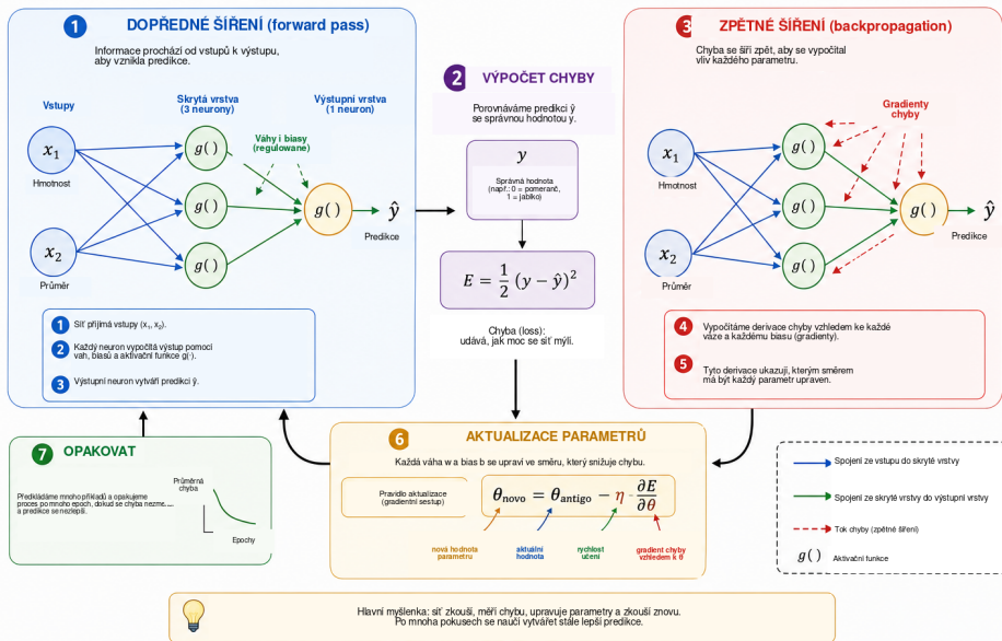
Obrázek 6: Základní cyklus tréninku neuronové sítě. Dopředné šíření převádí vstupy na predikci; ztrátová funkce měří rozdíl mezi predikcí a cílovou hodnotou; zpětné šíření počítá gradienty pomocí řetězového pravidla; a gradientní sestup tyto gradienty používá k aktualizaci vah a biasů. Opakování tohoto cyklu po mnoho epoch nazýváme učením.
