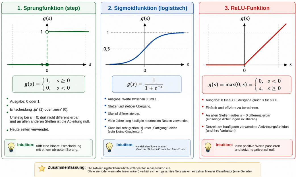
Abbildung 4: Vergleich dreier Aktivierungsfunktionen, die häufig in einführenden Darstellungen neuronaler Netze verwendet werden. Die Sprungfunktion trifft eine abrupte Entscheidung; die Sigmoidfunktion liefert einen glatten Übergang zwischen 0 und 1; und ReLU unterdrückt negative Eingaben, während positive erhalten bleiben. Nichtlineare Aktivierungen verhindern, dass eine Folge von Schichten zu einer einzigen affinen Transformation zusammenfällt.
