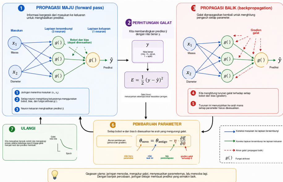
Gambar 6: Siklus dasar pelatihan jaringan saraf. Propagasi maju mengubah masukan menjadi prediksi; fungsi galat mengukur ketidaksesuaian antara prediksi dan target; propagasi balik menghitung gradien dengan aturan rantai; dan penurunan gradien menggunakan gradien tersebut untuk memperbarui bobot dan bias. Pengulangan siklus ini selama banyak epoch adalah proses yang kita sebut pembelajaran.
