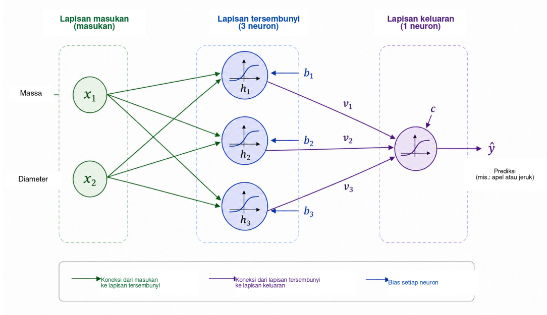
Gambar 5: Arsitektur didaktis 2–3–1 yang digunakan untuk memperkenalkan komputasi jaringan saraf. Dua masukan — massa dan diameter — diberikan kepada tiga neuron pada lapisan tersembunyi. Aktivasi h_1, h_2, h_3 kemudian digabungkan oleh neuron keluaran untuk menghasilkan prediksi \hat{y} . Setiap koneksi memiliki bobot yang dapat disesuaikan dan setiap neuron memiliki bias.
