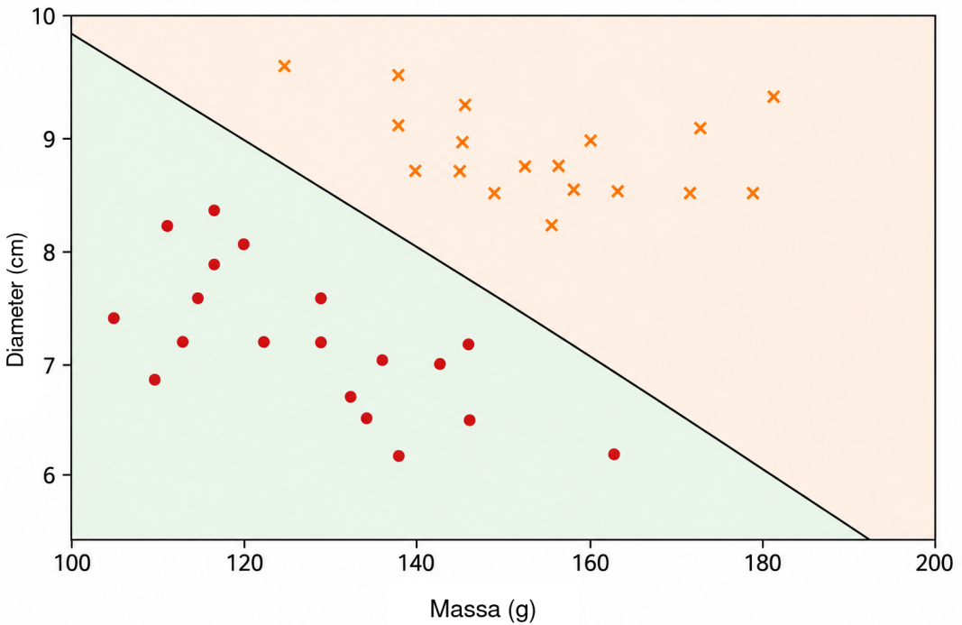
Gambar 2: Contoh pengklasifikasi linear pada bidang massa–diameter. Garis lurus bertindak sebagai batas keputusan: titik-titik pada satu setengah bidang menerima satu kelas, sedangkan titik-titik pada setengah bidang yang berlawanan menerima kelas lainnya. Karena itu, keputusan hanya bergantung pada sisi garis tempat titik tersebut berada.
