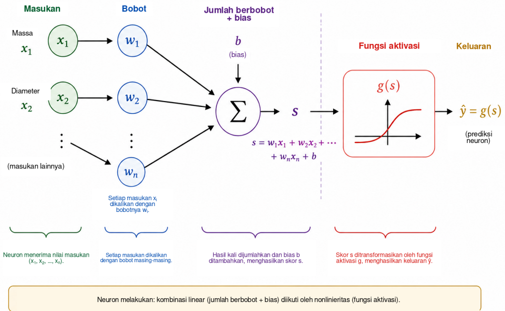
Gambar 3: Skema kerja neuron tiruan. Setiap masukan x_i dikalikan dengan bobot w_i ; hasil-hasil kali dijumlahkan dengan bias b untuk menghasilkan skor s . Fungsi aktivasi g kemudian mengubah skor ini menjadi keluaran \hat{y} = g(s) , yang dapat digunakan sebagai besaran antara atau sebagai prediksi akhir.
