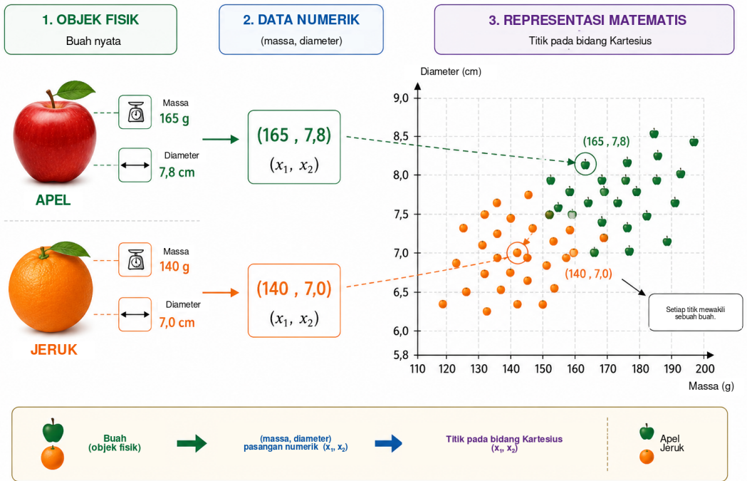
Gambar 1: Dari pengamatan fisik ke pemodelan matematis. Setiap buah mula-mula dideskripsikan oleh dua besaran terukur — massa dan diameter — lalu direpresentasikan oleh pasangan terurut (x_1, x_2) . Pada bidang massa–diameter, setiap pengamatan menjadi sebuah titik, sehingga membedakan apel dari jeruk dapat ditafsirkan kembali sebagai masalah geometri untuk memisahkan dua kelas.
